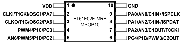
图 1-5 MSOP10 (A)
