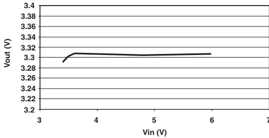
Vout Vs. Vin* Iout = 0.1A
