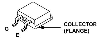
JEDEC TO-263AB
