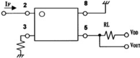
G3VM-61FR, -61FR(TR)
