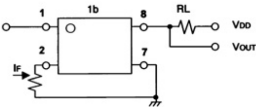
G3VM-355FR, -355FR(TR)
