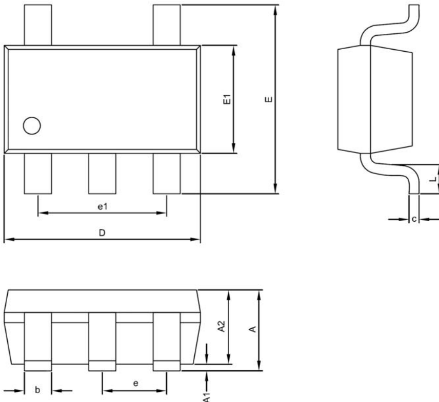
SOT-23-5 Package
