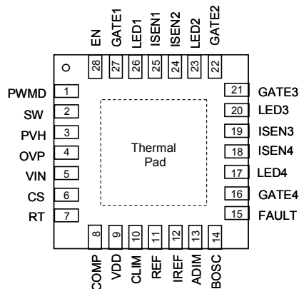
G5996A TQFN4X4-28
