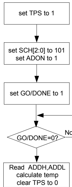
温度计量
