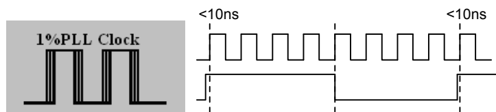
PLL 误差
