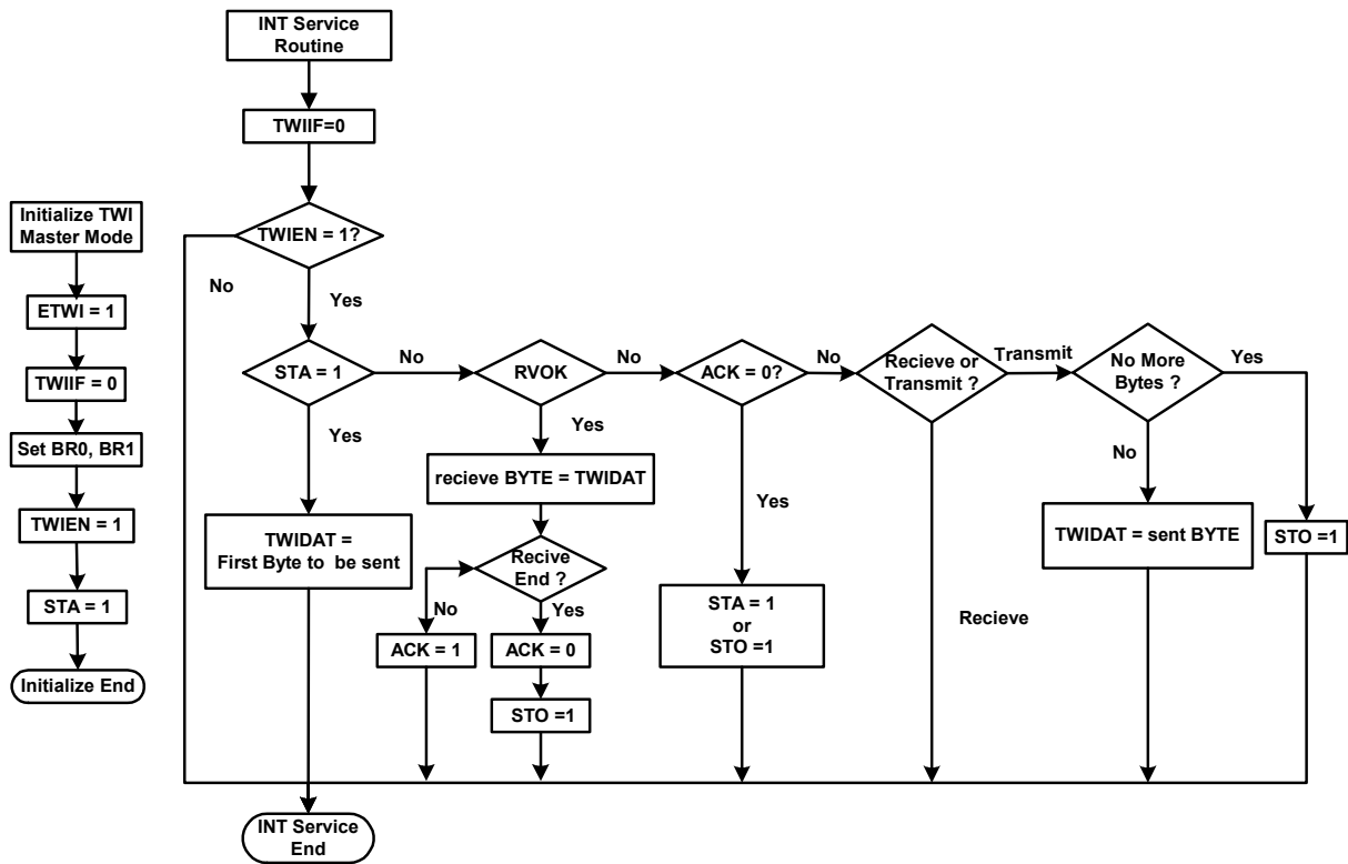
软件流程图
