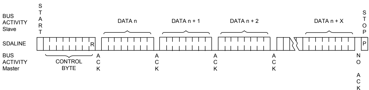
主接收模式的数据传输
