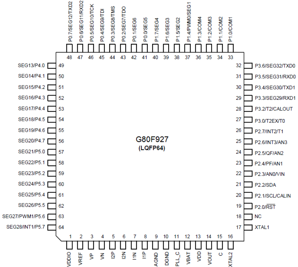
引脚配置图
