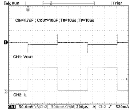
Load Transient(G965-15)
