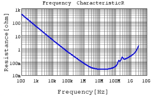
GC321AD72E103KX01 R DCOV, 25degC
