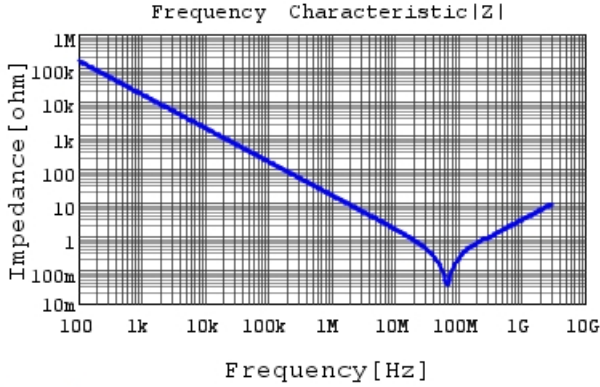
GC321AD72E103KX01 |Z| DCOV, 25degC
