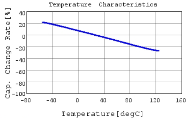
GC321AD72E103KX01 C-Temp. capchange, DCOV, 1
