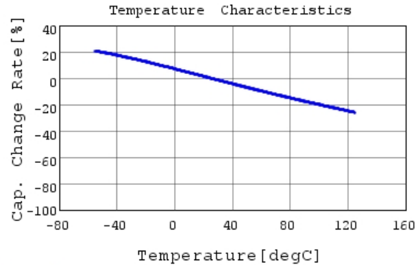
GC331AD72W103KX01 C-Temp. capchange, DCOV, 1
