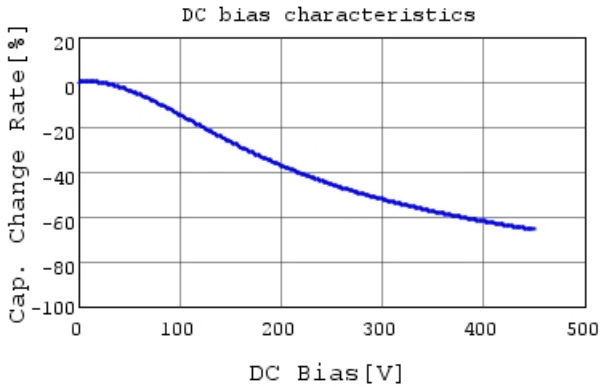
GC331AD72W103KX01 C-DC bias capchange, 25.0c
