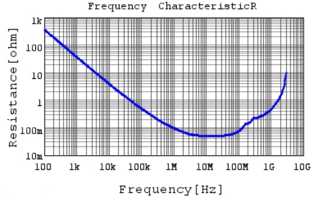
GC331AD72W103KX01 R DCOV, 25degC
