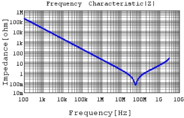
GC331AD72W103KX01 |Z| DCOV, 25degC
