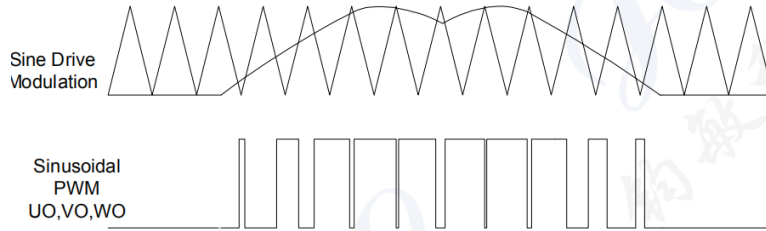
Sinusoidal PWM
