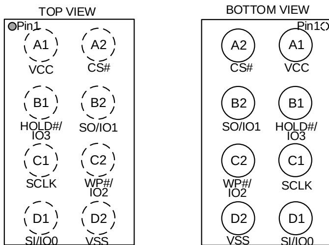
WLCSP
