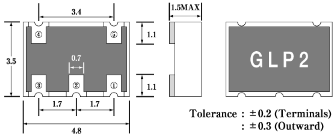
Dimension (Unit : mm)
