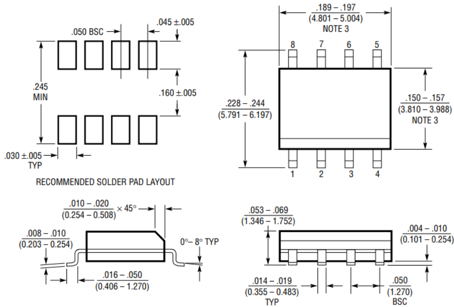
图 21.5 引脚 SOP-8
