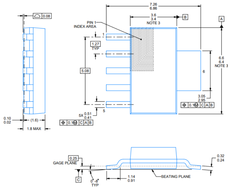
图 22.5 引脚 TO-263
