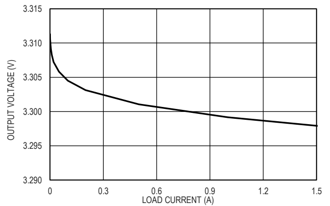
图 9. 3.3V 输出电压和负载电流的关系
