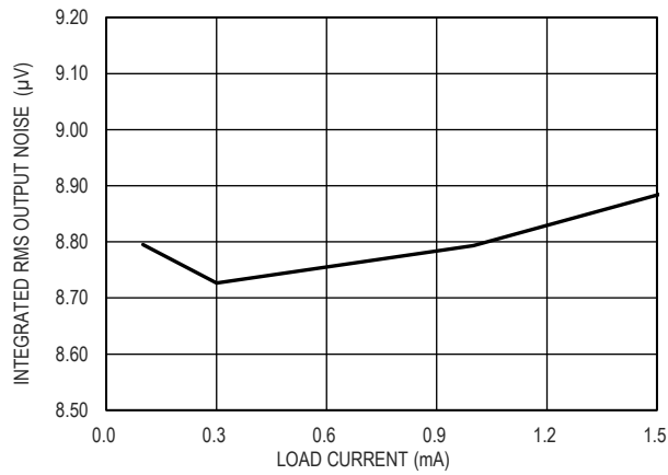
图 16. 积分 RMS 输出噪声, V_{IN}=5V , V_{OUT}=3.3V
