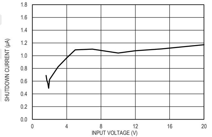
图 7. 关机电流和输入电压的关系
