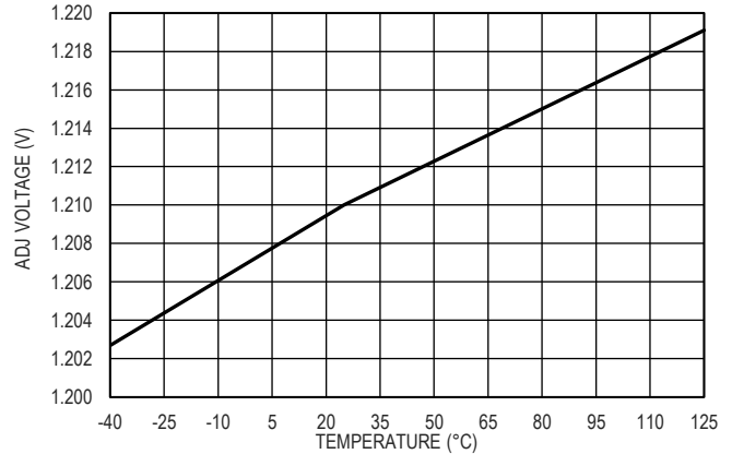
图 11. ADJ 引脚电压精度
