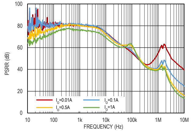
图 17. 电源电压纹波抑制比, V_{IN}=5V , V_{OUT}=3.3V
