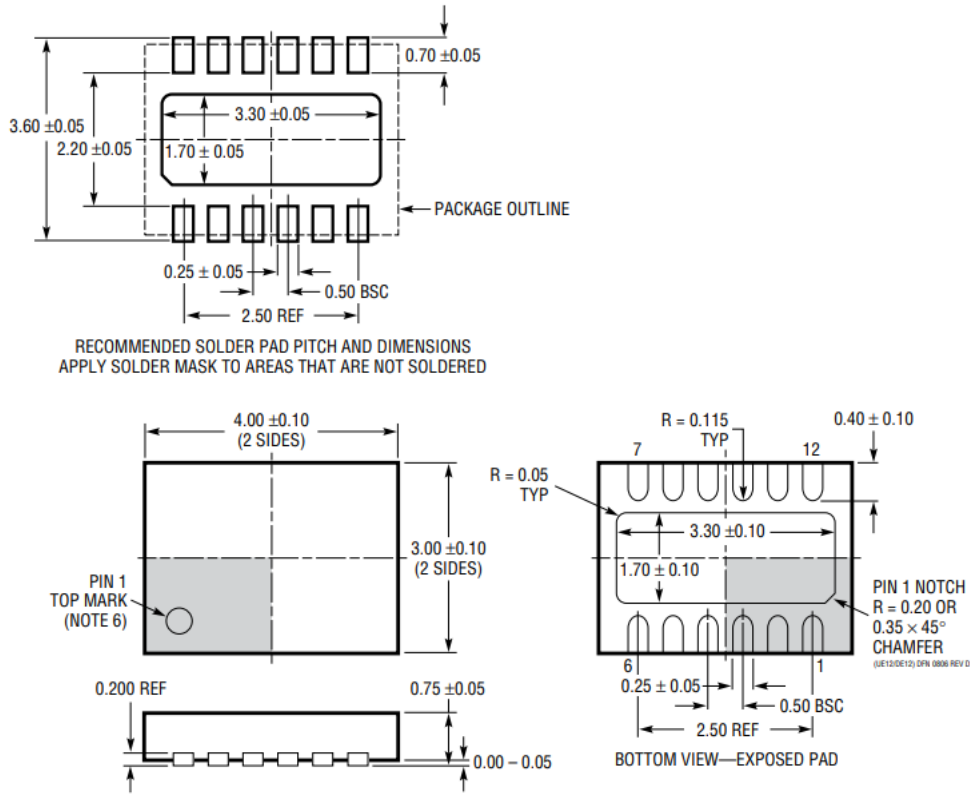
图 22. 16 引脚 TSSOIC
