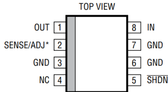
8 引脚 SOIC 图 2 引脚配置
