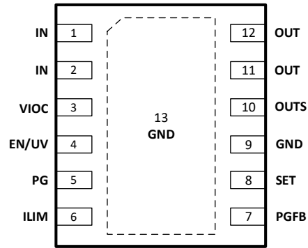
图 3. 引脚配置(顶视图)
