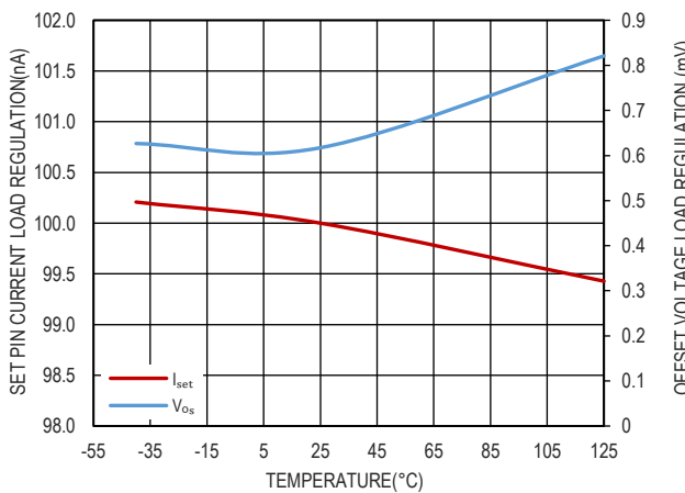
图 8. SET pin 电流温度的关系
