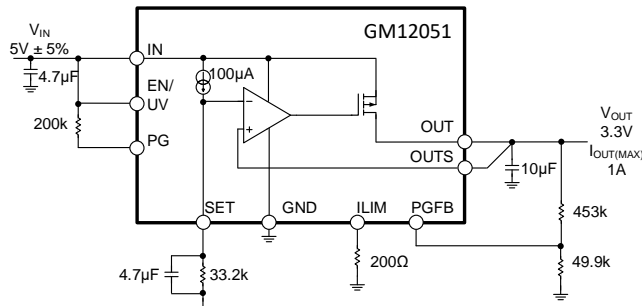
图 22 典型应用
