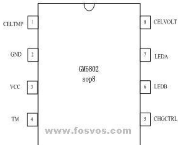
图 1 GM6802 引脚排布图
