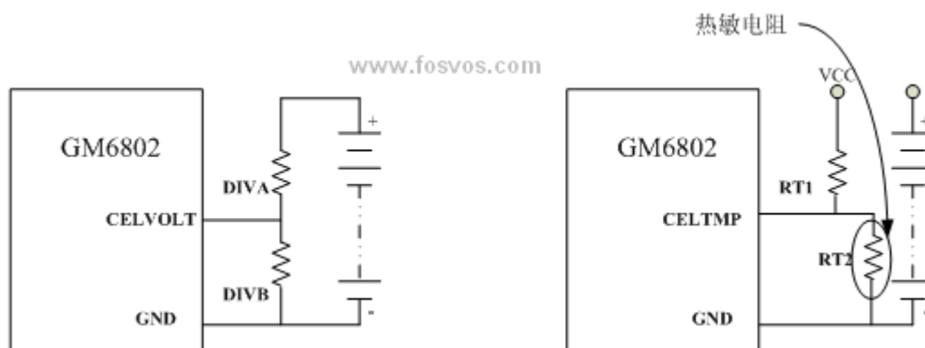
图 2 电池电压和温度检测原理图
