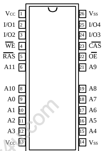
24(26) SOJ
