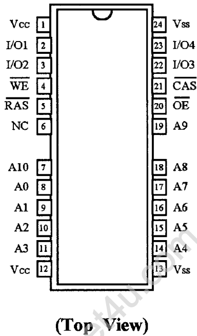
24 (26) SOJ
