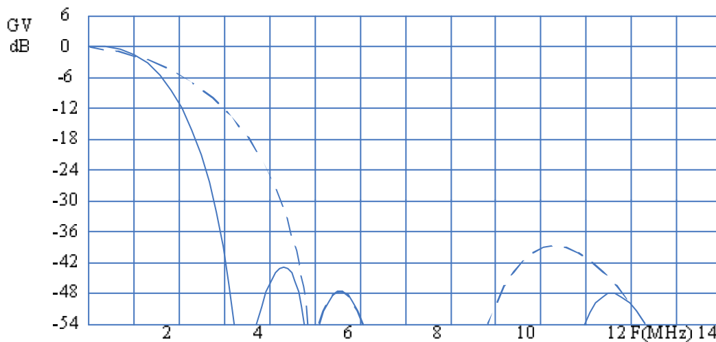
图表 3 色度滤波器频谱图
