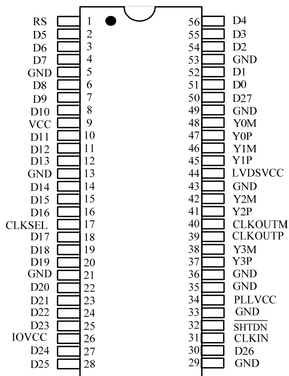
图 1 TSSOP56 引脚排布图
