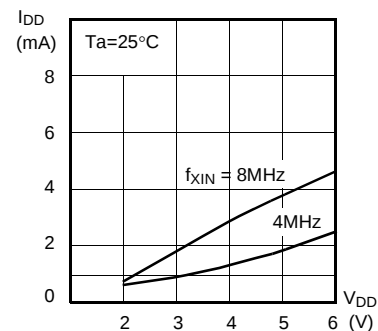
I_{DD}-V_{DD}
