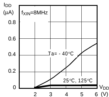
I_{STOP}-V_{DD}
