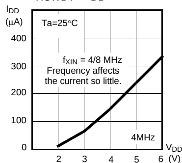
I_{RCWDT}-V_{DD}
