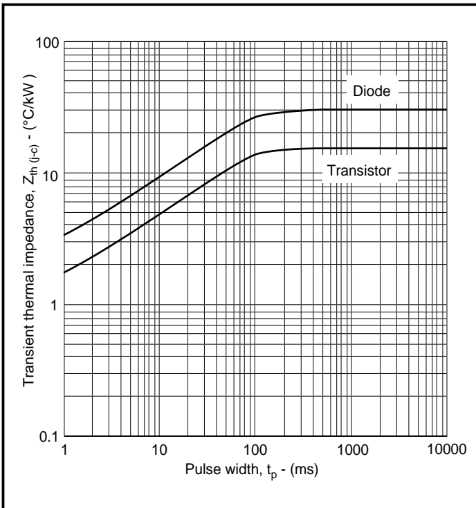
Fig. 9 Transient thermal impedance
