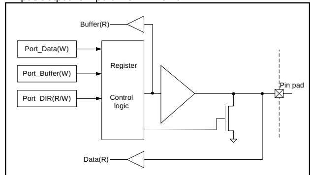
Input/Output IOC port : IOC7 - IOC0
