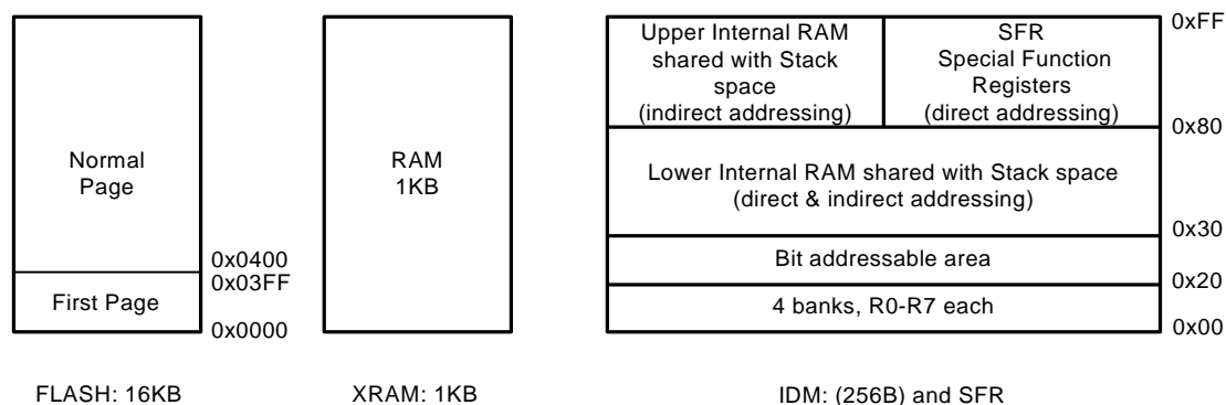
图 5-1 程序存储区和数据存储器
