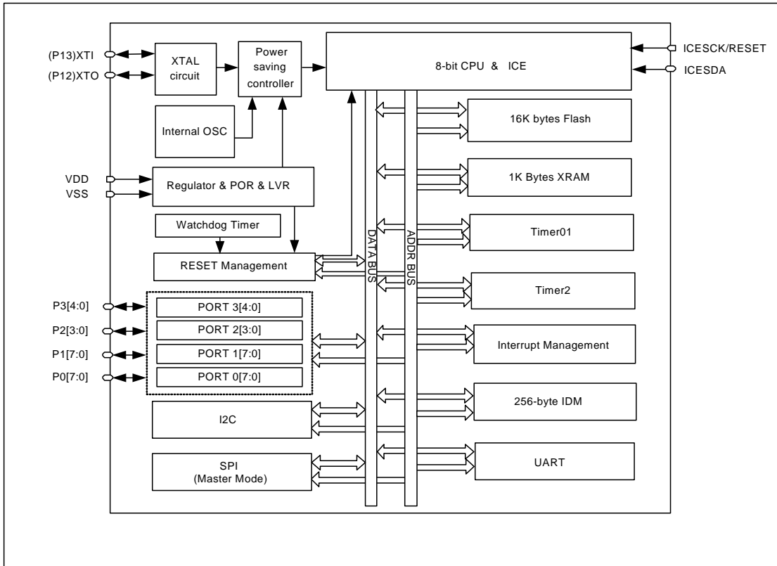
图 3-1 GPM8F3716B 框图
