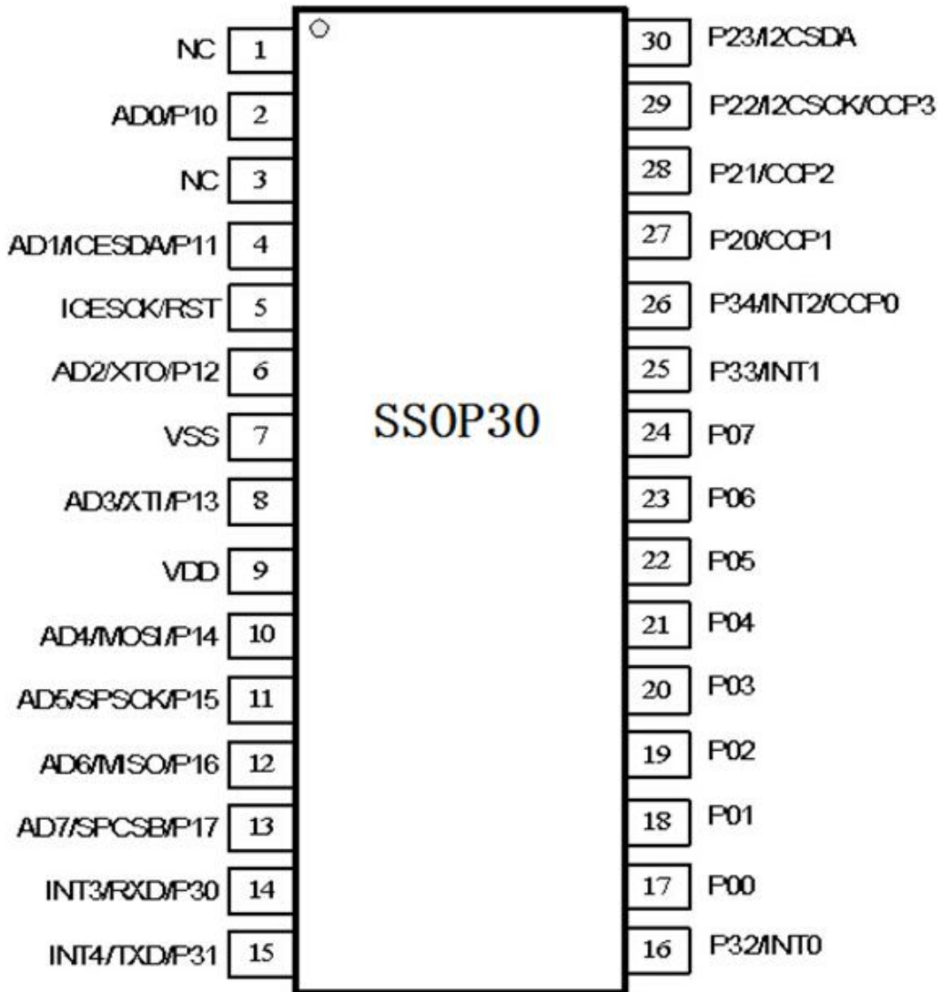
图 4-2 GPM8F3716B(SSOP30)脚位图
