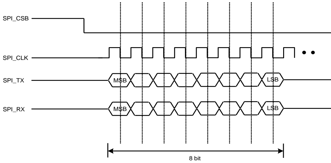
图 5-27 主模式，POLARITY=0，PHASE=1
