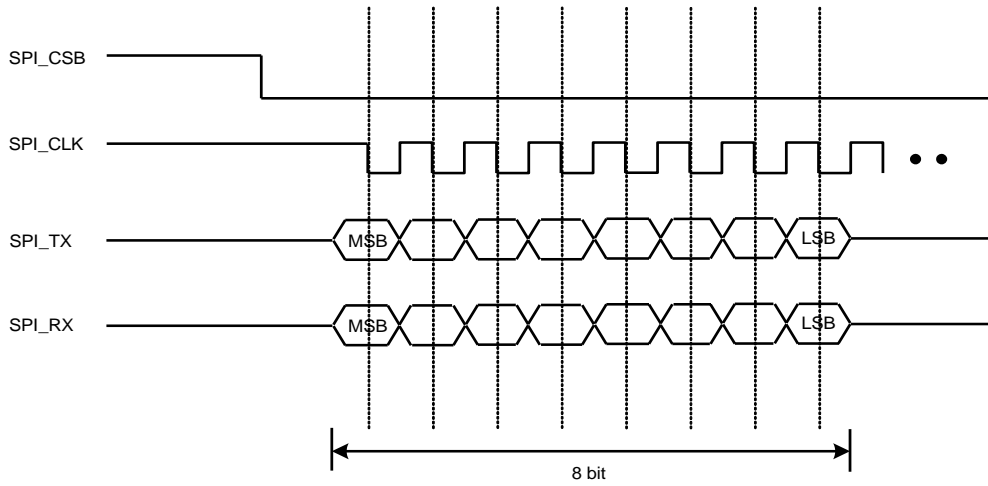
图 5-28 主模式，POLARITY=1，PHASE=0
