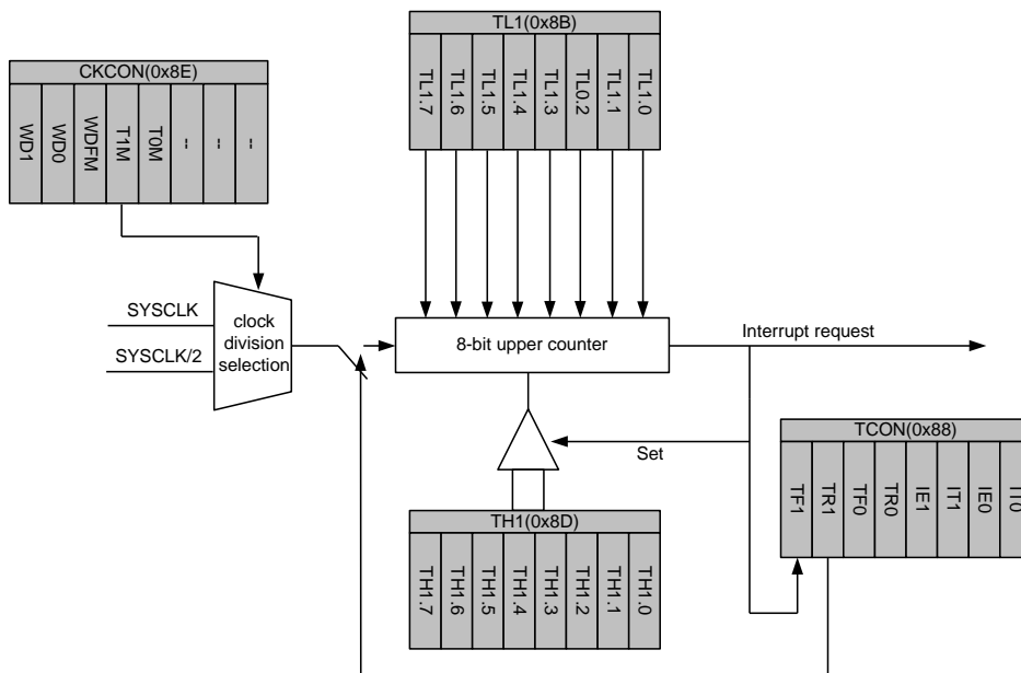
图 5-16 Timer 1 模式 2 示意图
