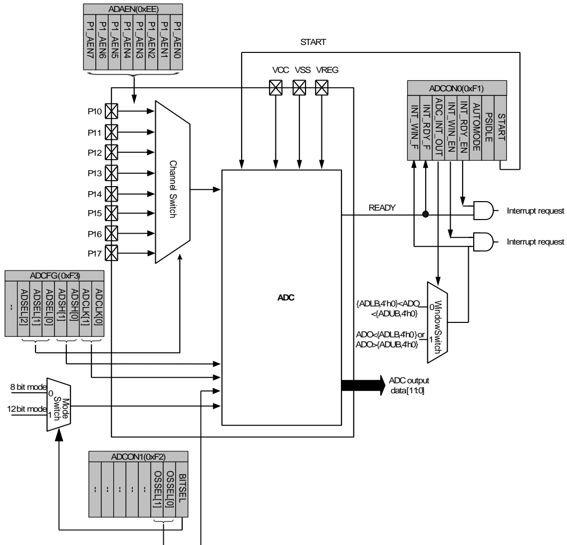
图 5-39 ADC 方框图
