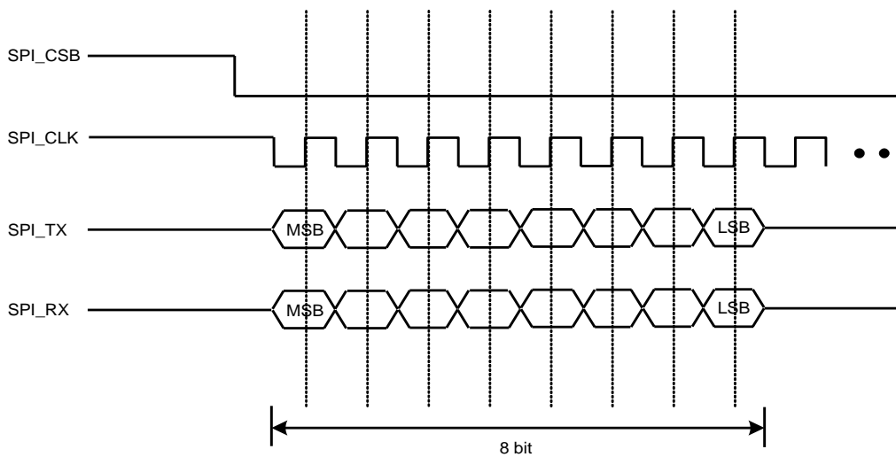
图 5-29 主模式，POLARITY=1，PHASE=1
