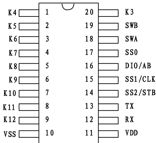
图5-1 GRM805_17 管脚图
