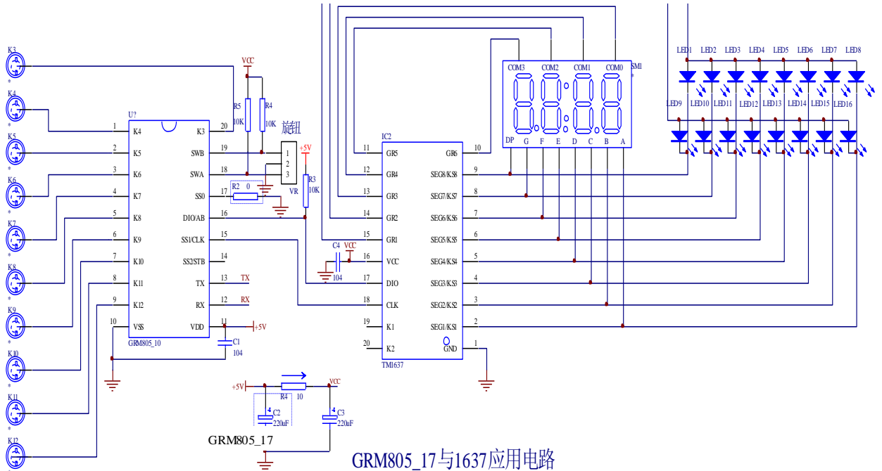
图6-2 GRM805_17触摸键配合1637显示应用电路
