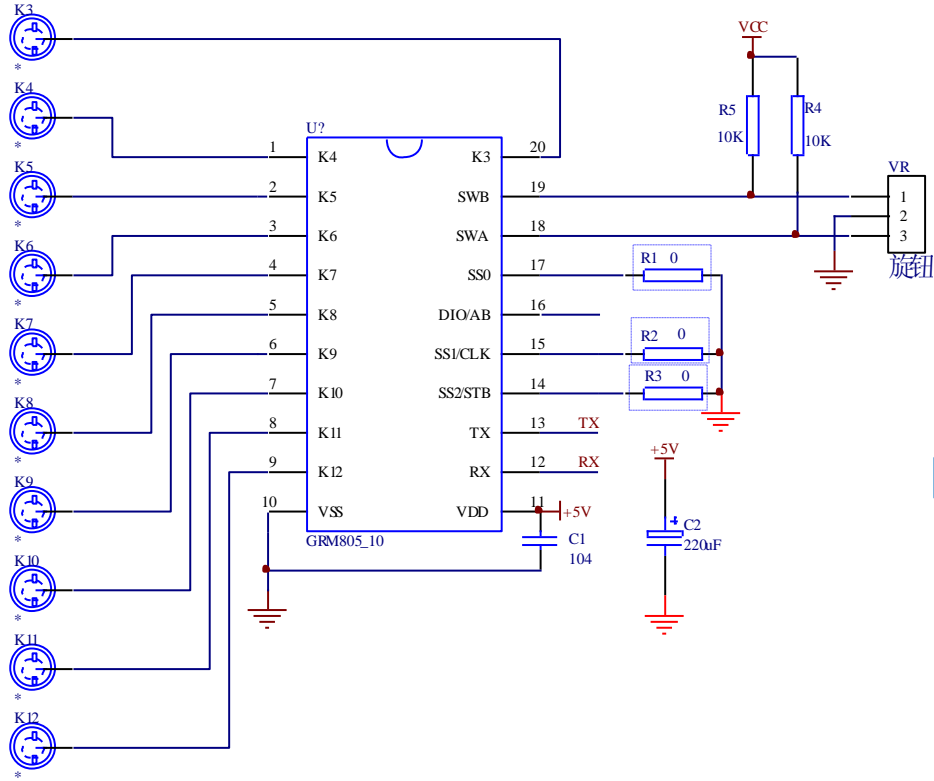
图 6-1 GRM805_17 作为纯触摸键应用电路
