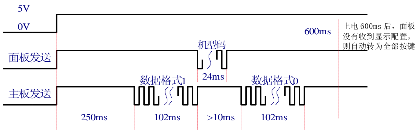
图 10-1 逻辑时序
