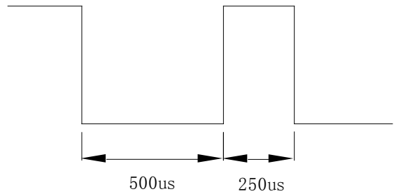
图 8-2 主板向面板发送“1”的定义
