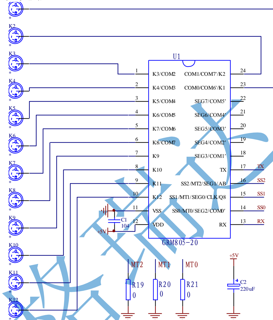
图6-1 GRM805_22作为纯触摸键应用电路
