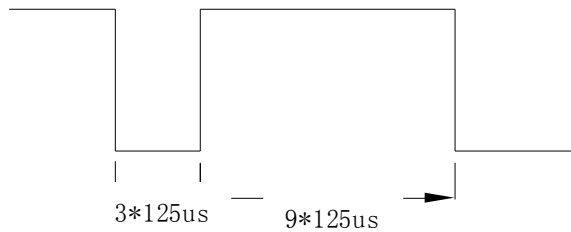
图 7-1 面板向主板发送 “0” 的定义
