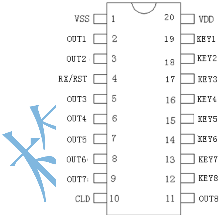
图5-1 GRM807FS_16 管脚图
