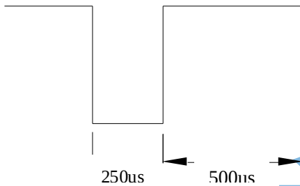
图 2-1 主板向面板发送“0”的定义
