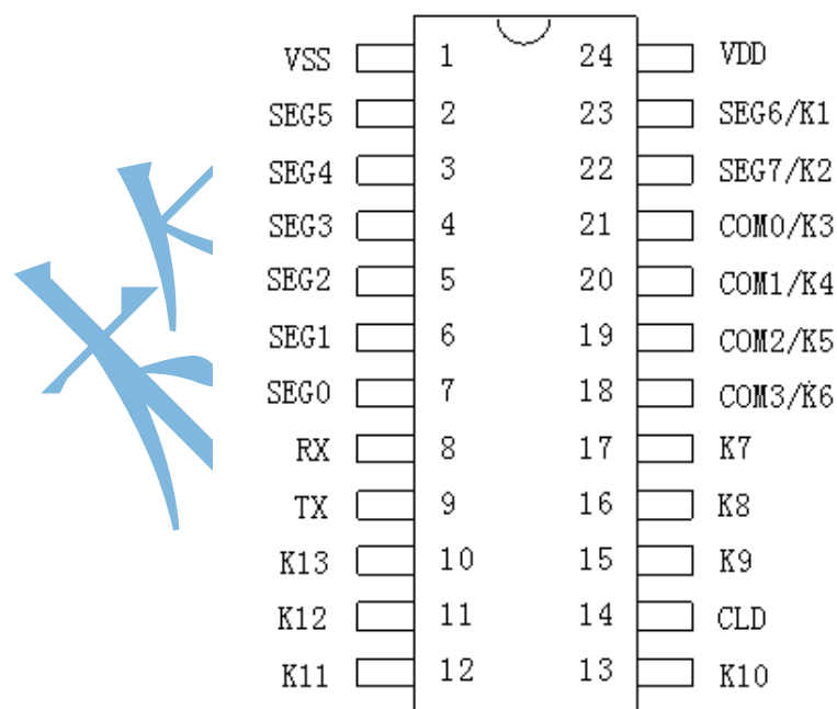
图 5-1 GRM808S_24 管脚图
