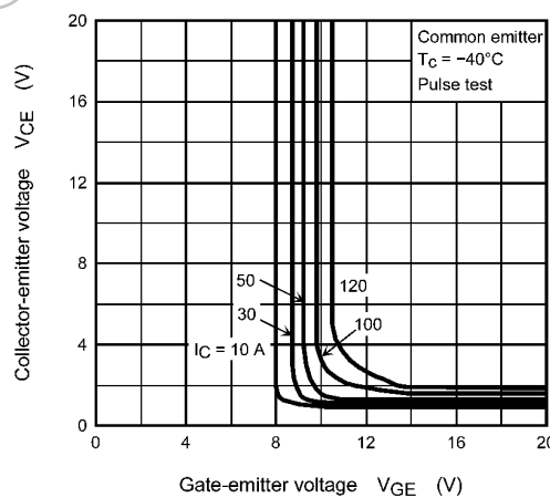
Fig. 8.6 V_{CE} - V_{GE}
