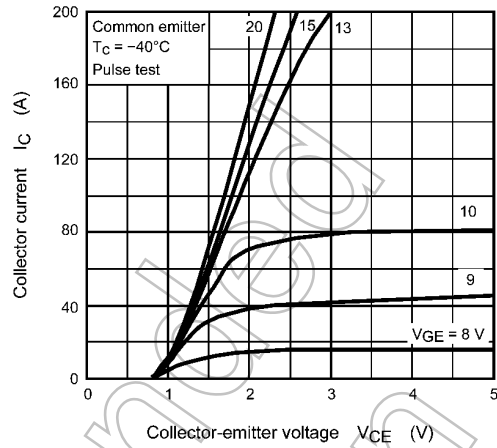
Fig. 8.2 I_C - V_{CE}
