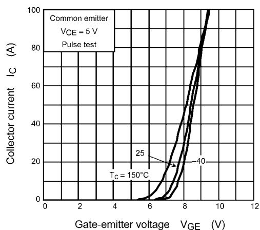
Fig. 8.6 I_C - V_{GE}
