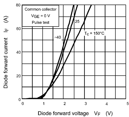
Fig. 8.13 I_F - V_F
