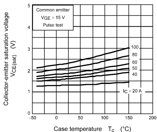
Fig. 8.5 V_{CE(sat)} - T_C
