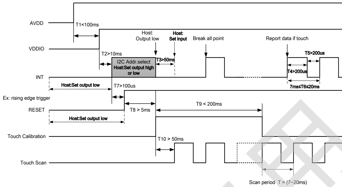
主控复位 GT970 时序图:
