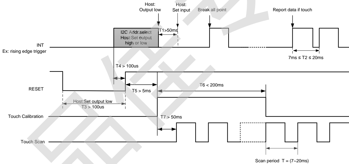
主控复位 GT970 时序图:
