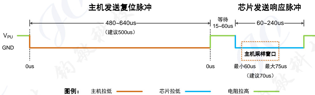
图 2. 初始化序列的时序图
