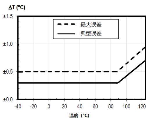
图 5 GXHT30 温度误差
