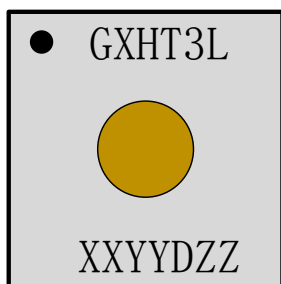
图 8 GXHT3L-DIS 顶视图以及激光标记
