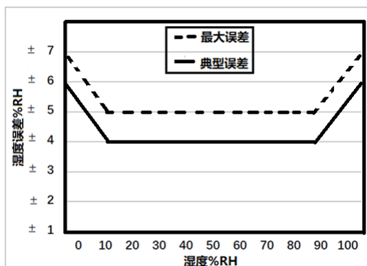
图 4 GXHT3L 湿度误差@25° C
