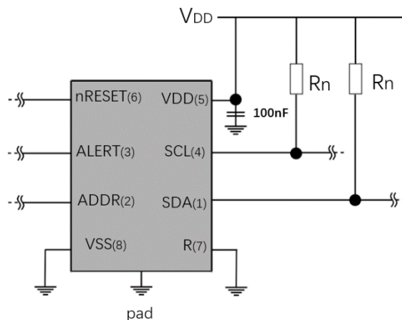
图 7 典型应用电路。需要注意图中的管脚位置只是示意图，和表 7 中的真实传感器管脚位置不同。
