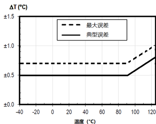
图 6 GXHT3L 温度误差
