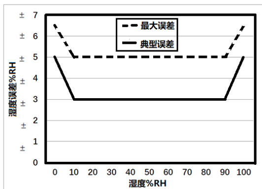
图 3 GXHT30 湿度误差@25° C
