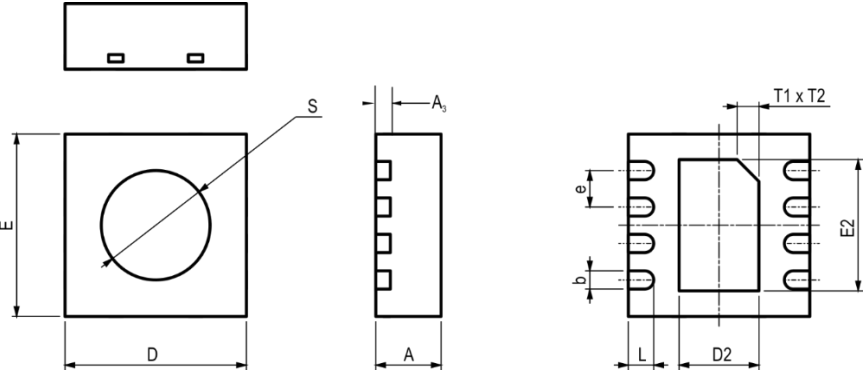
图 9 GXHT3L-DIS 传感器封装尺寸
