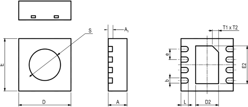
图 14 GXHT3L 传感器封装尺寸
