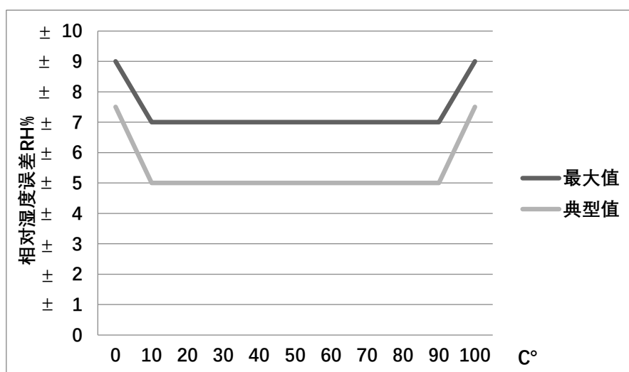
图 3 GXHT3L 在 25 摄氏度下的相对湿度误差 (%RH)
