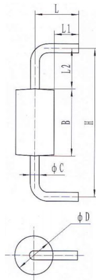
DO-201AD-B1 成型图及尺寸
