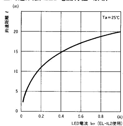
■到達距離/LED電流特性 \ell/I_{FP}
