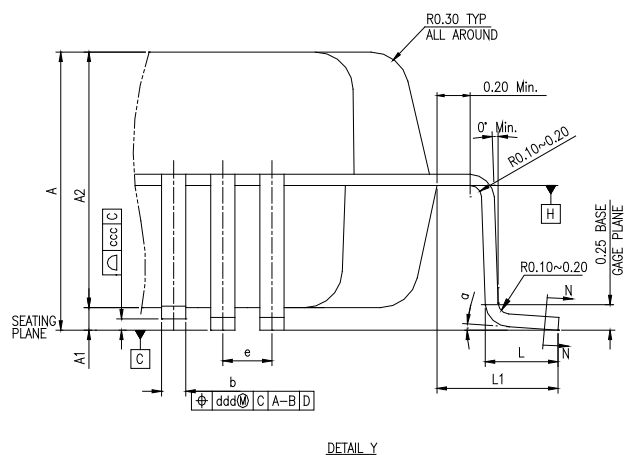
DETAIL Y
