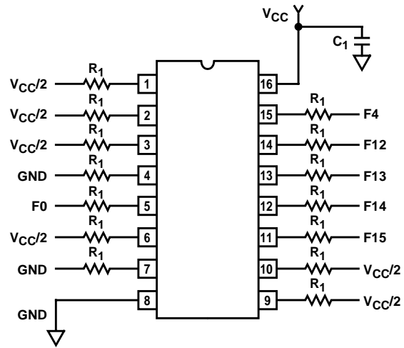
HD-4702/883 CERDIP
