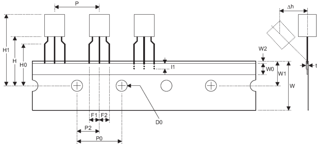
TO92
