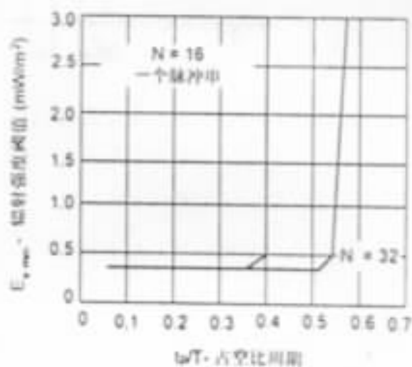
图2. 灵敏度和占空比周期
