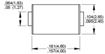
DO-214AC (SMA)
