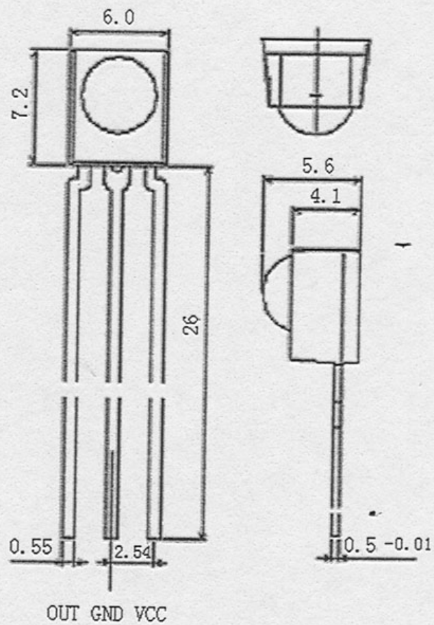
外型尺寸及引脚排列：
