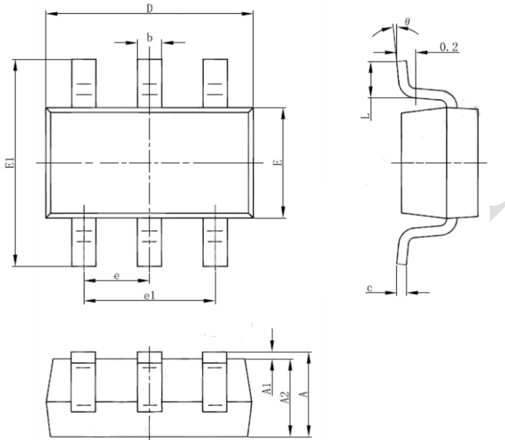
SOT-23-6 封装外观图
