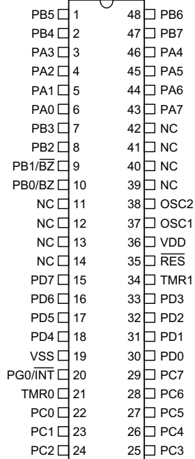
HT48E50 – 48 SSOP-A
