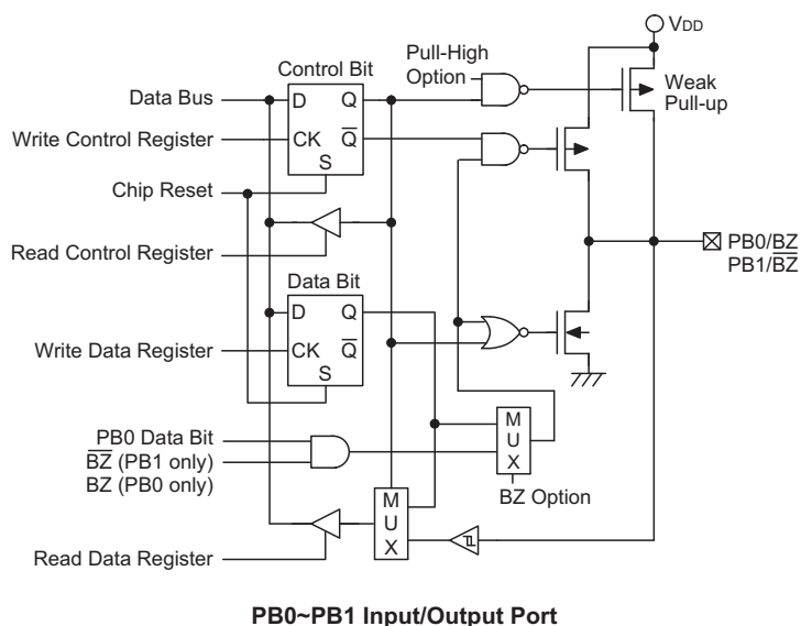
PB0~PB1 Input/Output Port
