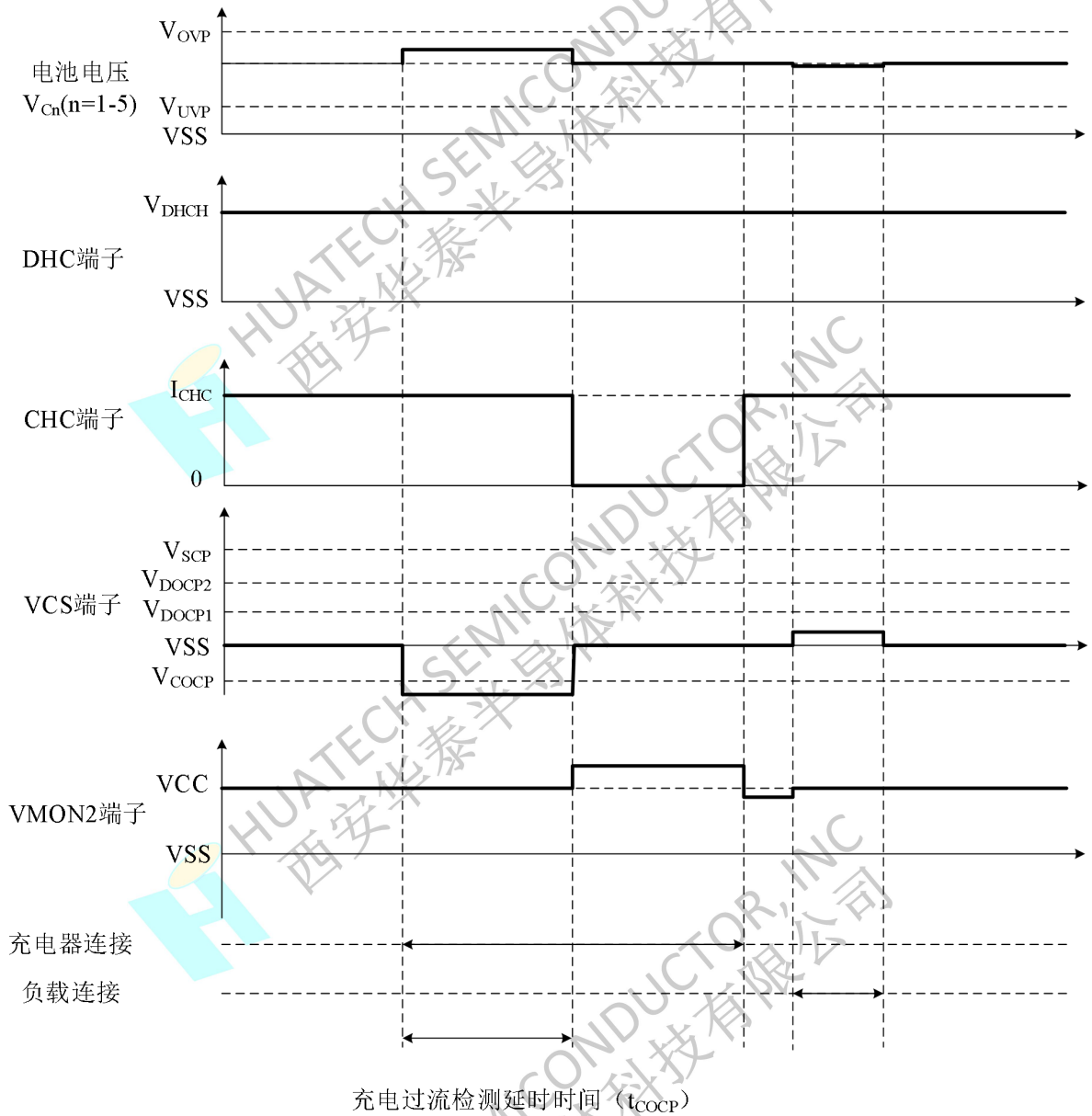
图 16 充电过流检测
