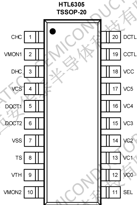
图7 引脚分布
