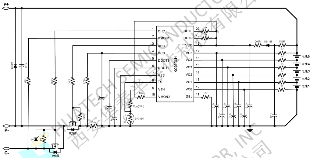
图 2 5 节电池包的 N 型充电管和 N 型放电管的 C-分口典型应用电路图
