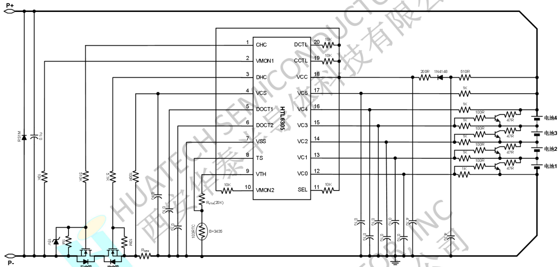
图 6 4 节电池包外部扩展均衡的 N 型充电管和 N 型放电管的同口典型应用电路图
