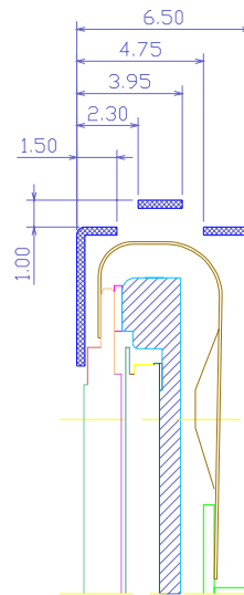
SECTION B-B(S:5/1)
