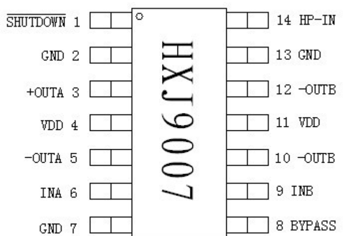
SOP-16
